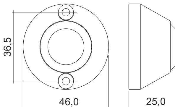
Obrázek 1. Rozměry zařízení
