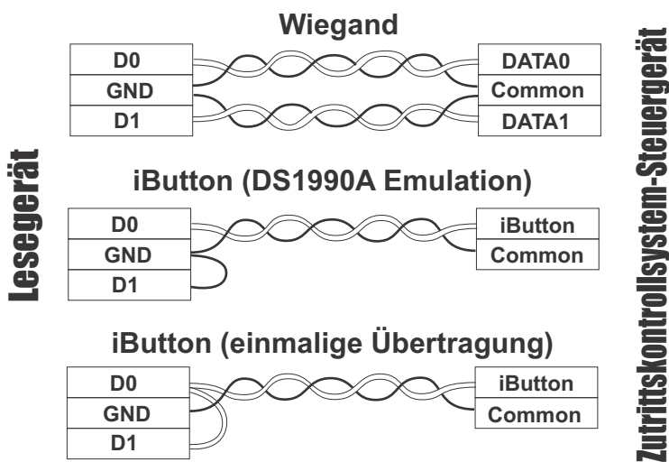
Abbildung 2. Auswahl des Übertragungsprotokolls.
