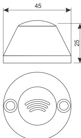
Abbildung 1. Geräteabmessungen.
