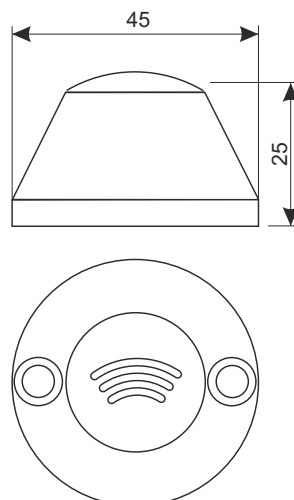
Figura 1. Medidas del dispositivo.
