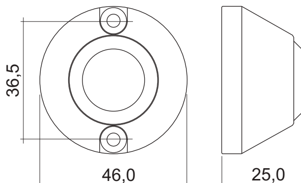
Figur 1. Enhetsdimensjoner.
